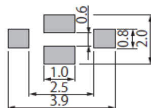
NFM3DCC/3DPC
