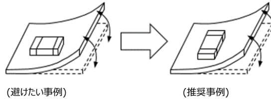
[ 部品方向 ]
