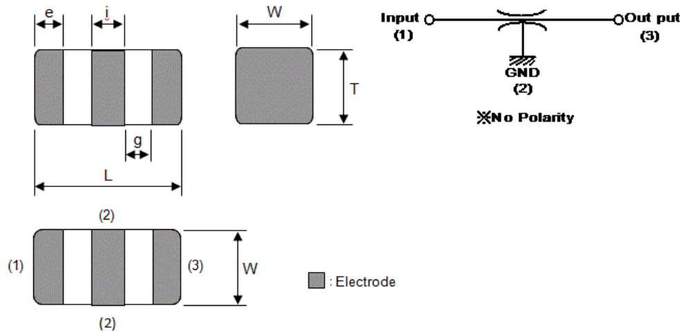
図: 寸法
