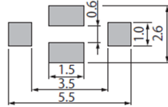
NFM41CC/41PC
