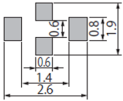
NFM21CC/21PC
