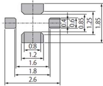
NFM21PS
