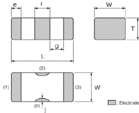
図:寸法
