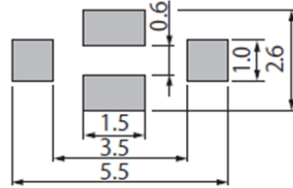
NFM41CC/41PC
