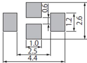
NFM31PC/31KC
