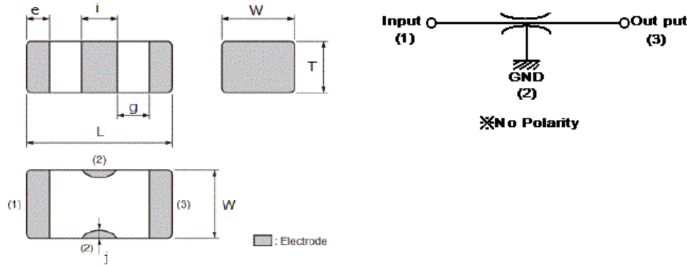
図:寸法
