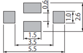
NFM41CC/41PC
