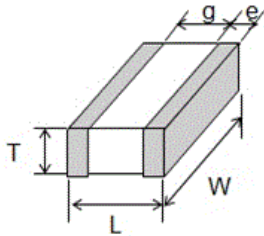
図:寸法
