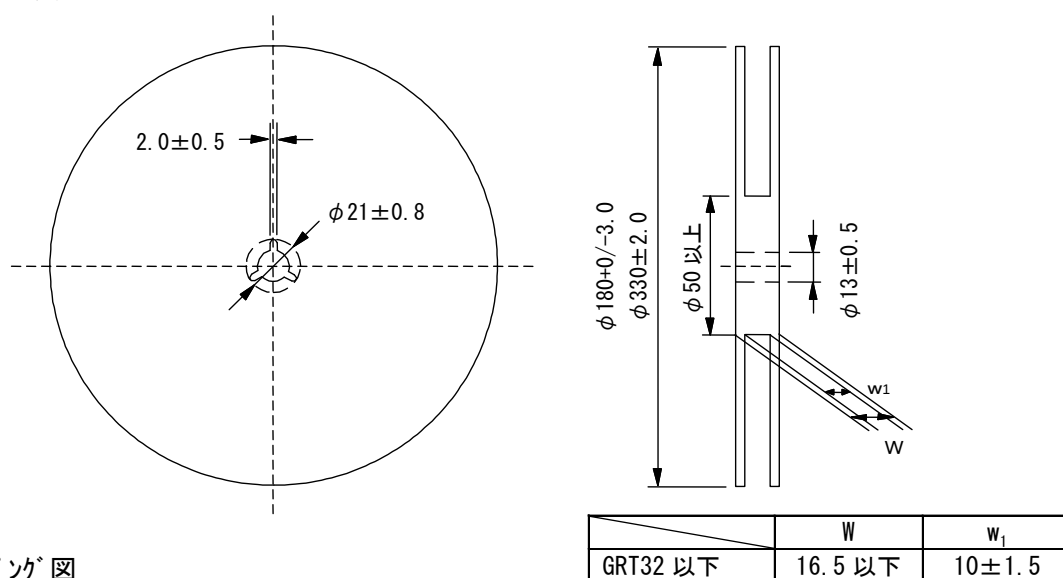
図2 リール寸法
