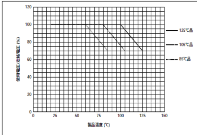
電圧・温度軽減(デレーティング)条件 (定格電圧100V以下品)
