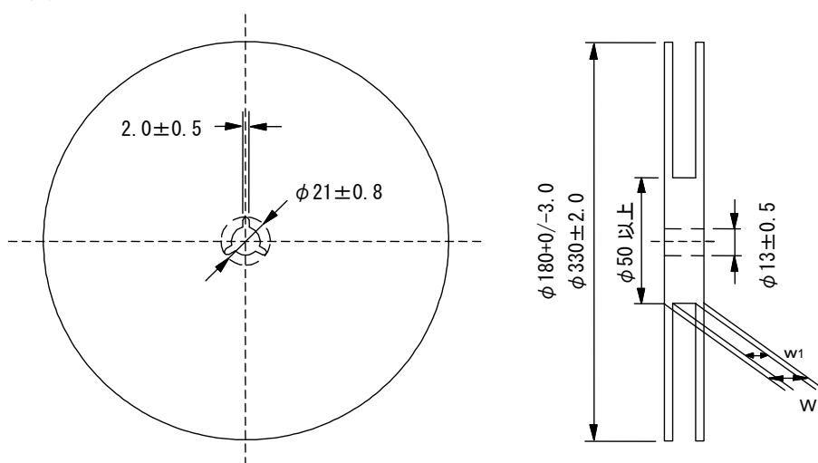
図2 リール寸法
