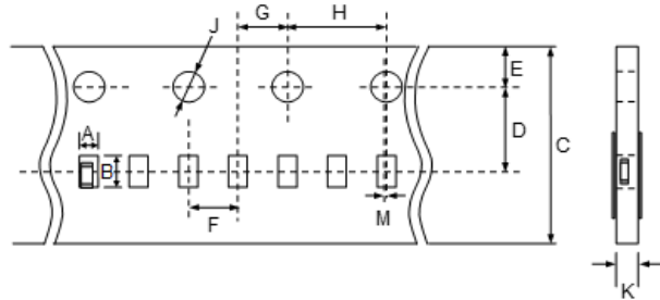
(1)GRT15(W8P2 包装記号 : D/J)
