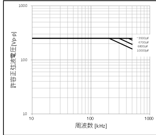
チップ(L×W):2.0×1.25mm COG(5C)特性、定格電圧:DC250V
