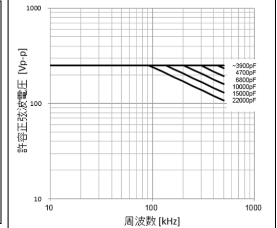
チップ(L×W):3.2×1.6mm COG(5C)特性、定格電圧:DC250V
