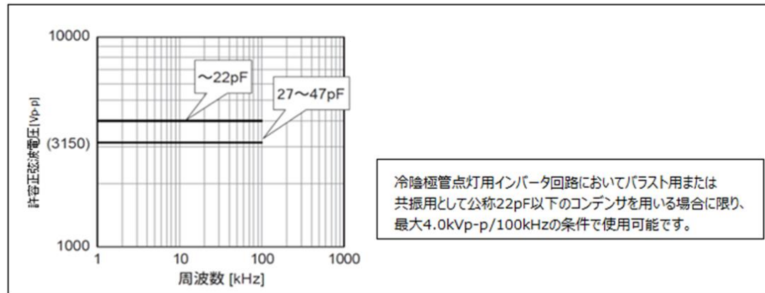
チップ(L×W):4.5×2.0mm COG(5C)特性、定格電圧:DC3.15kV
