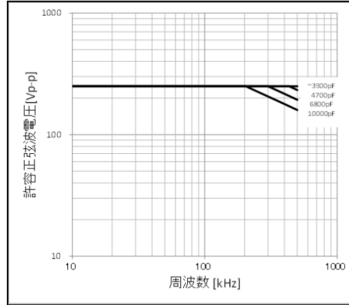
チップ(L×W):2.0×1.25mm COG(5C)特性、定格電圧:DC250V
