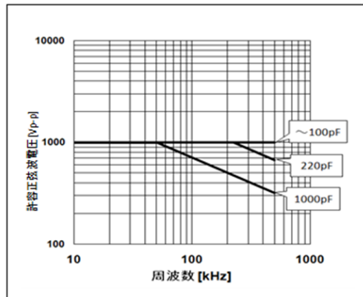
チップ(L×W):3.2×1.6mm COG(5C)特性、定格電圧:DC1kV
