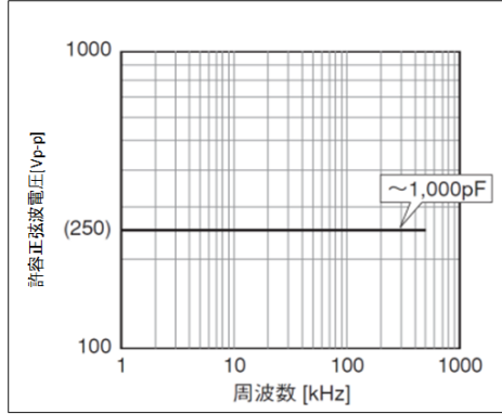
チップ(L×W):1.6×0.8mm COG(5C)特性、定格電圧:DC250V
