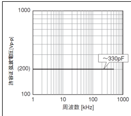
チップ(L×W):2.0×1.25mm COG(5C)特性、定格電圧:DC200V
