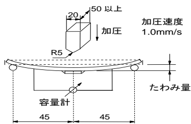
図2 (単位:mm)
