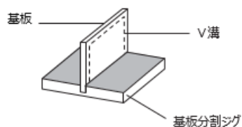
[ ジグ概要 ]
