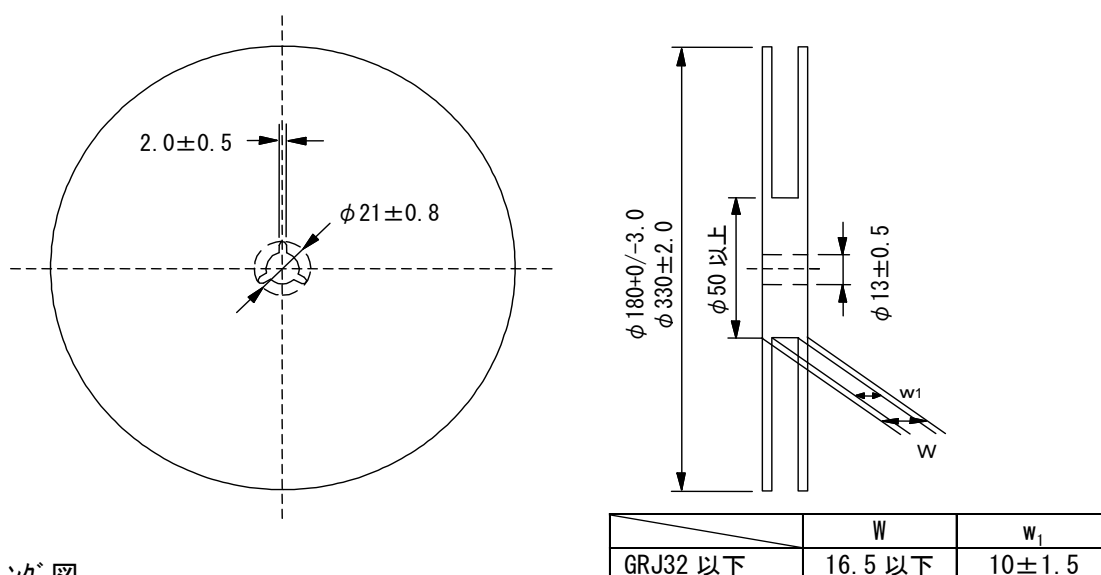
図2 リール寸法
