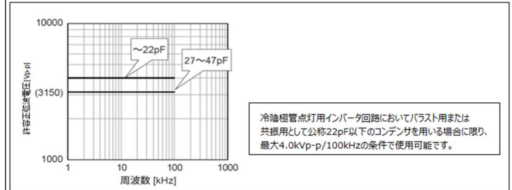
チップ(L×W):4.5×2.0mm COG(5C)特性、定格電圧:DC3.15kV
