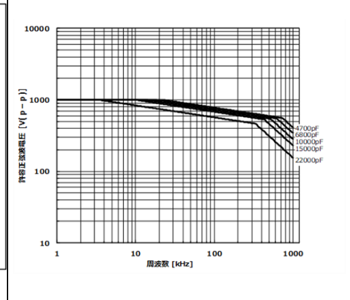
チップ(L×W):3.2×2.5mm COG(5C)特性、定格電圧:DC1kV
