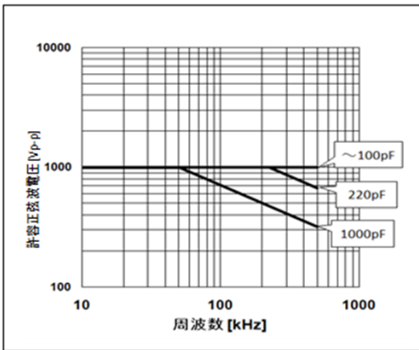
チップ(L×W):3.2×1.6mm COG(5C)特性、定格電圧:DC1kV
