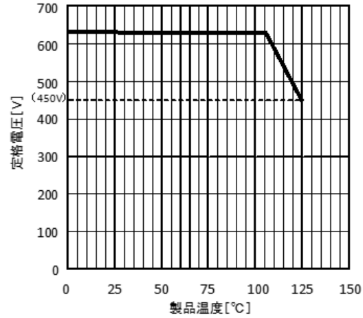
図: 定格電圧デレージング
