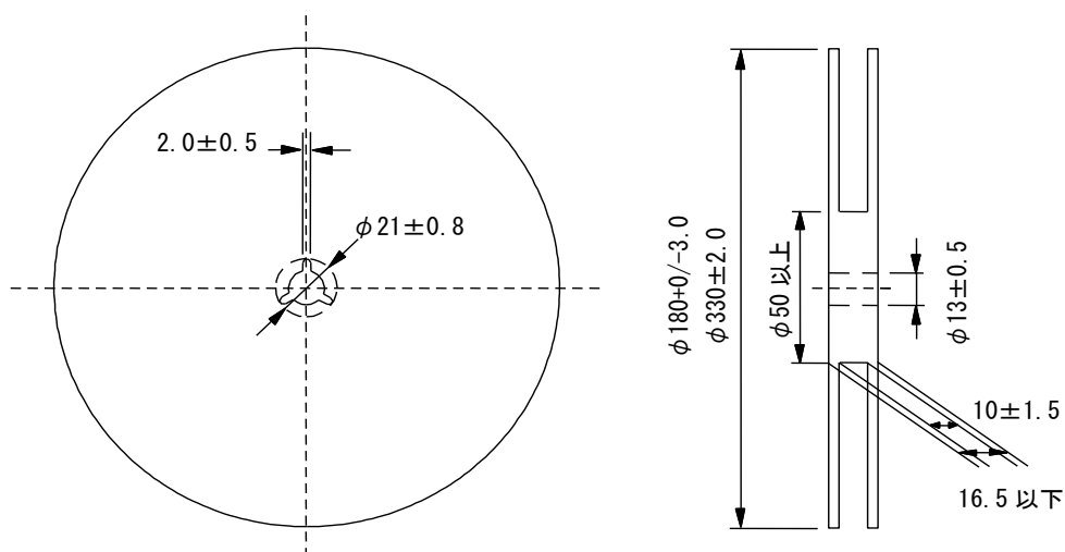
図2 リール寸法図
