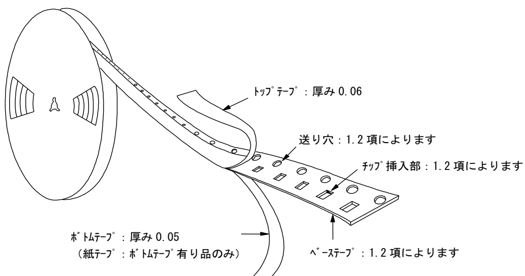
図3 テーピング図
