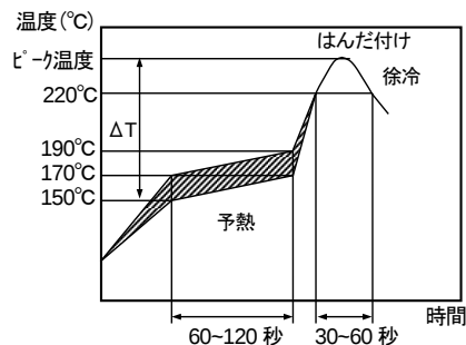
[リフローはんだ付け許容温度、時間]
