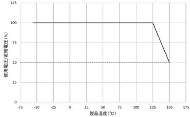
図: 定格電圧デレーティング
