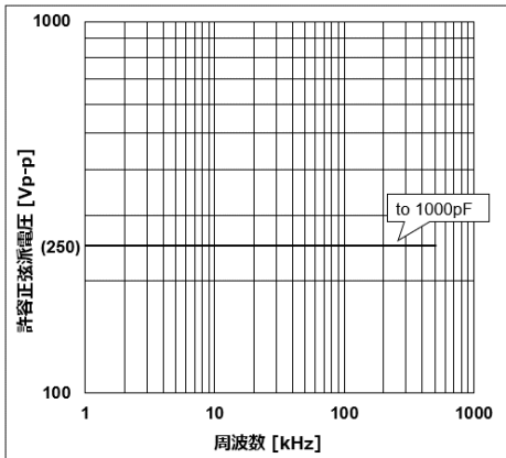
チップ(L×W):1.0×0.5mm C0G(5C) 特性、定格電圧:DC250V
