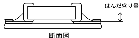
断面図
