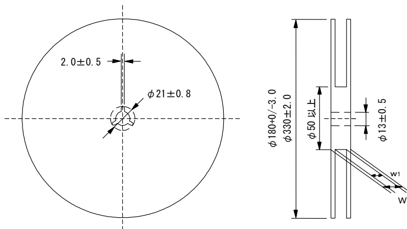
図2 リール寸法
