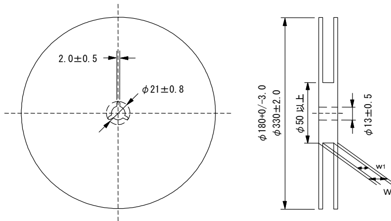
図2 リール寸法
