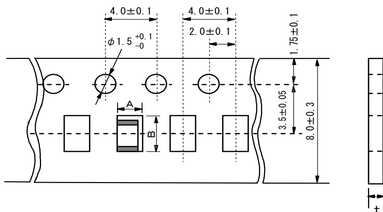
(2) GCJ18/GCJ21 <紙テープ>
