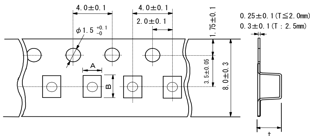
(3) GCJ21/GCJ31/GCJ32 <プラスチックテープ>
