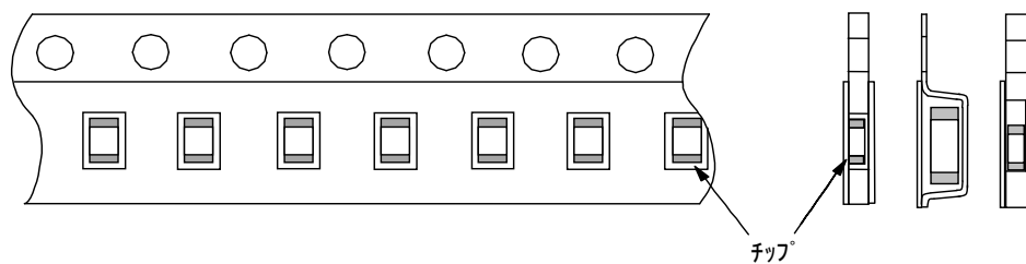
図1 チップ詰め状態
