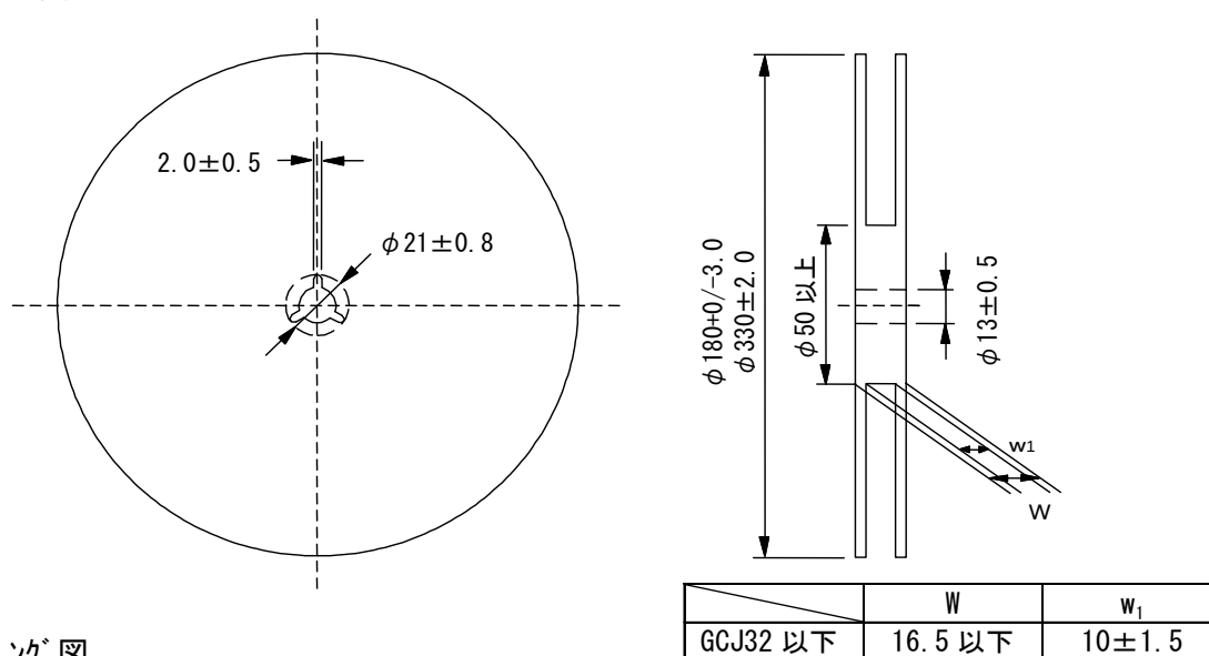
図2 リール寸法
