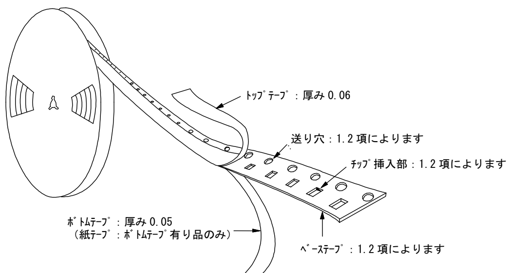
図3 テーピング図
