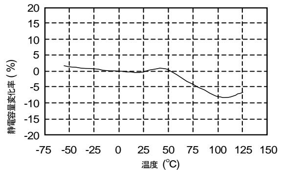
□ 静電容量 - 温度特性 R7特性の例
