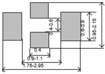
NFM18HC106
