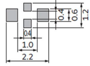
NFM18CC/18PC* *Except for NFM18PC106.
