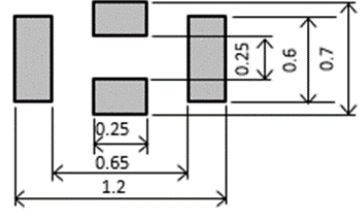
NFMJMPL
