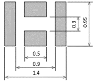
NFM18HC105
