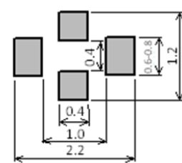
NFM18HC105
