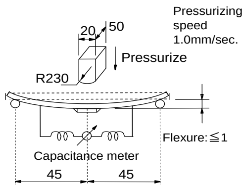
Fig.2 (in:mm)
