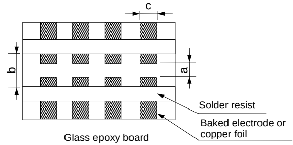
Fig.3 (in:mm)
