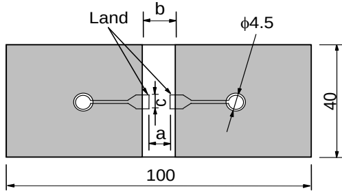
Fig.1 (in:mm)
