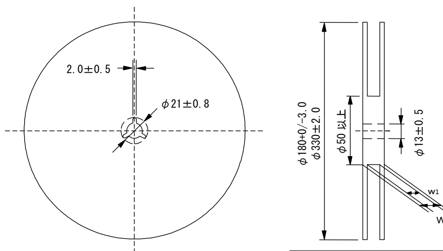
図2 リール寸法
