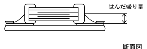
断面図
