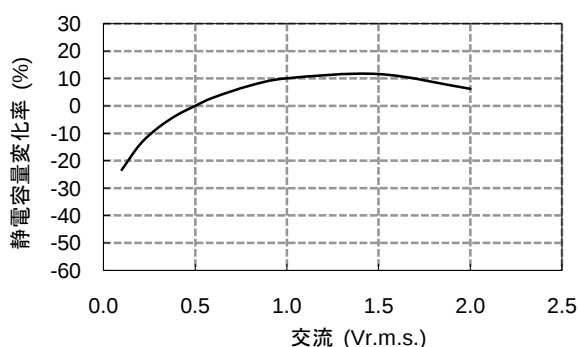
□ 交流電圧特性の例
