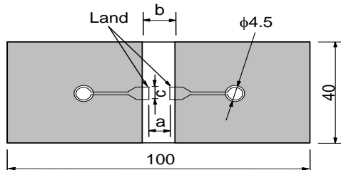
Fig.1 (in:mm)
